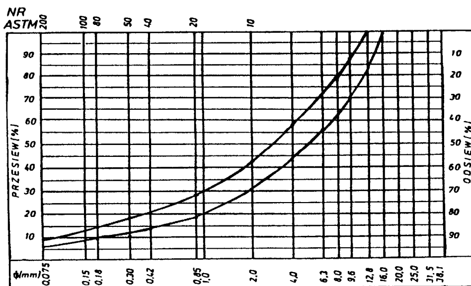
Rys. 6. Krzywe graniczne uziarnienia mieszanki mineralnej 0+16 mm do warstwy ścierniej z betonu asfaltowego dla KR 3-6
