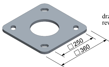
PODSTAWA 1
